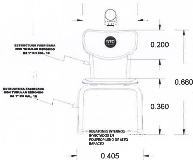
ALZADO FRONTAL
