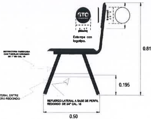
ALZADO LATERAL
