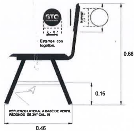
ALZADO LATERAL
