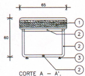
CORTE A - A'.
